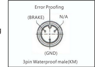
彥豪W19海因(公)3pin 接腳定義圖
